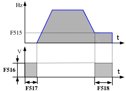
图 9-2 直流制动
