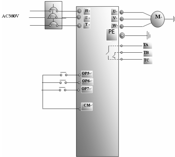
图 4-2 接线图 2
